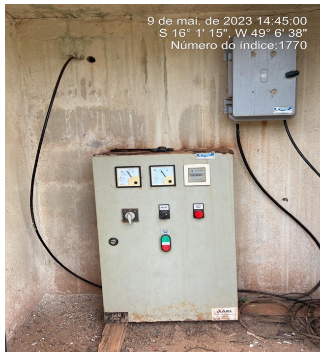
Foto 4 - Poço P2 com pintura desgastada do abrigo do quadro de comando e sem aviso de risco.
